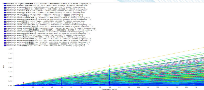
图 3-20 混合标准线性溶液谱图
