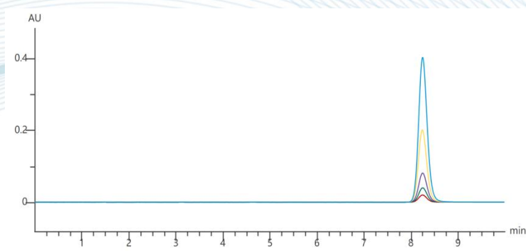
图 1-23 标准线性溶液谱图
