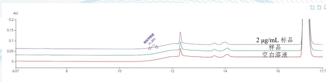
图 1-18 实际样品色谱图
