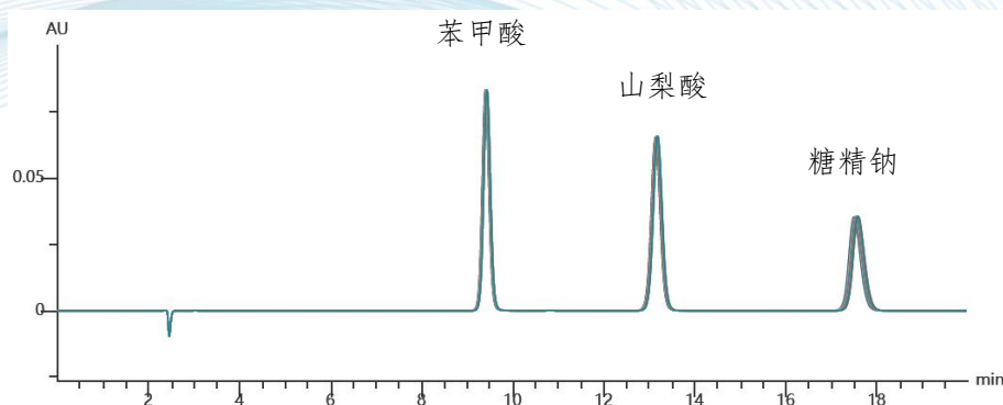
图 1-1 混合标准溶液重复性谱图 (n=6)
