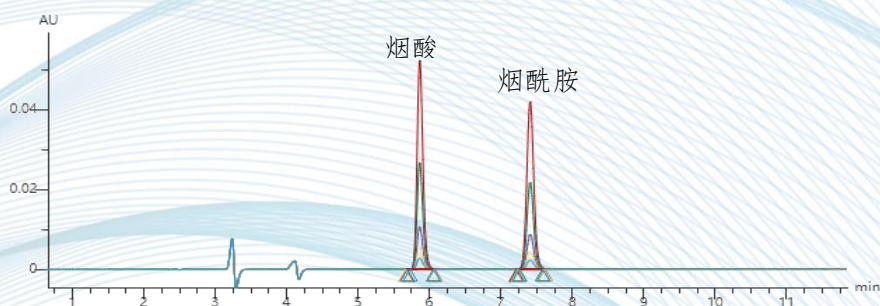
图 2-12 混合标准线性溶液谱图
