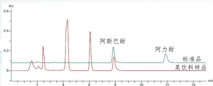
图 1-16 实际样品色谱图
